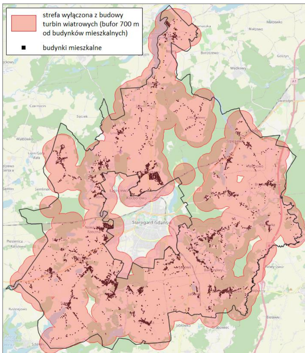
Rysunek 15. Orientacyjny obszar wyłączony z lokalizacji elektrowni wiatrowych na terenie Gminy Starogard Gdański (bufor 700 m od budynków mieszkalnych)
